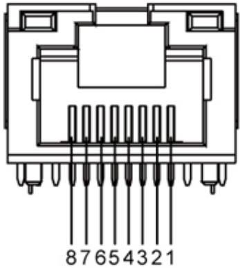
Разводка контактов разъема RJ45 для 10BASE-T и 100BASE-TX
